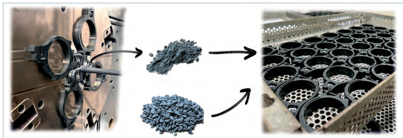
Kreislaufführung des Angussverlusts durch Zerkleinerung, Beimischung zu Neuware und direkte Rückführung. © Fraunhofer ICT
